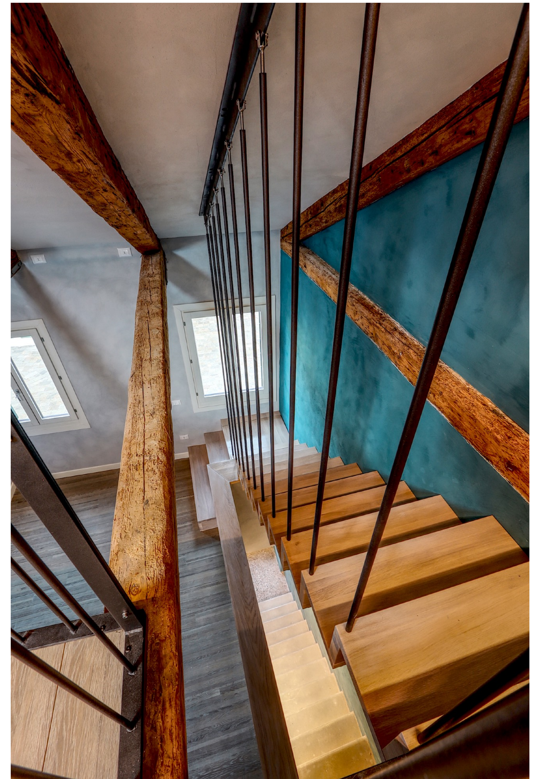
la scala appesa al tetto tramite dei tiranti e occhielli in acciaio appositamente realizzati uno ad uno per adeguarsi alle irregolarità strutturali tipiche dell'architettura veneziana
